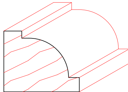
TM6025 1-1/16" X 1-1/16"
