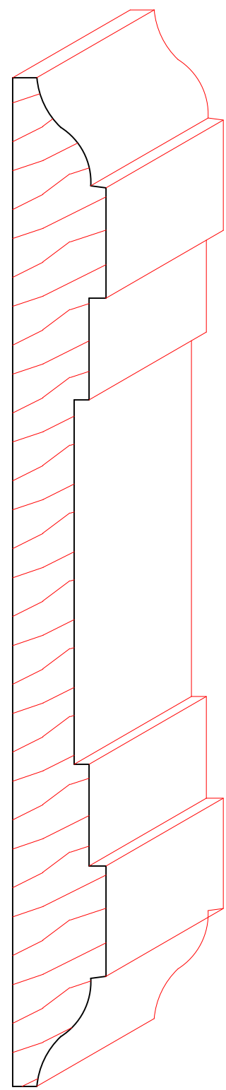
TM6053 11/16" x 7-7/16"
