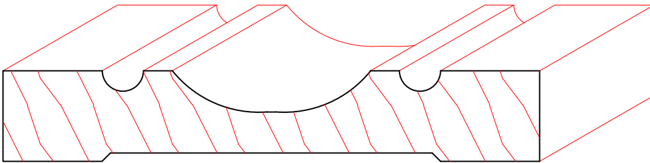
TM1035 11/16" X 4-1/16"
