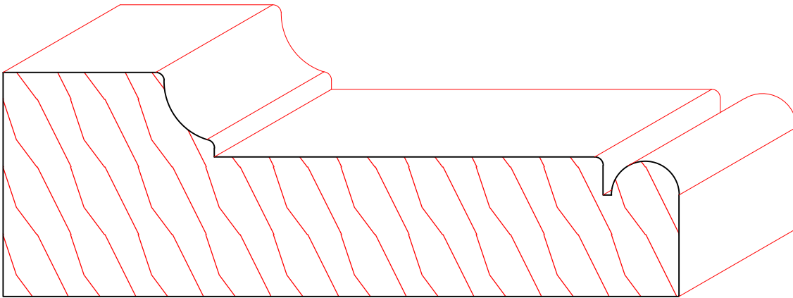
TM1251 1-11/16" X 5"
