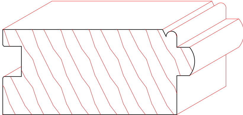
TM8009 1-1/2" X 3-3/8" +-
