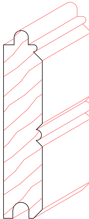
TM8003 11/16" X 3-5/16" +-
