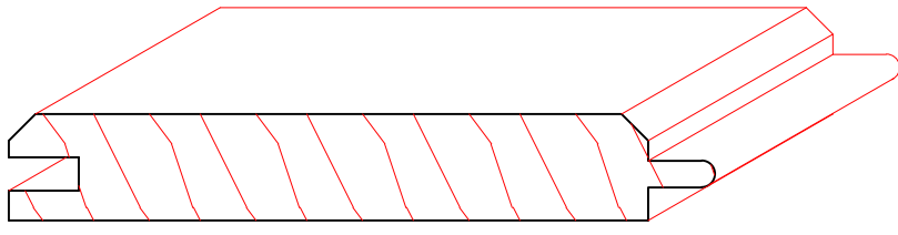
TM8020 1/2" X 3-5/16" +-
